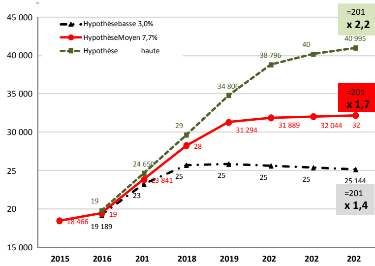
Figure 14 : Prévisions de la production en 2022 (MWh)
